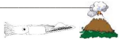
Belemnit
